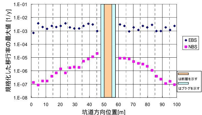
断層と坑道の交差点部にプラグを設置したケース
