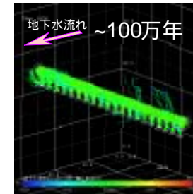
3次元核種移行解析における粒子軌跡の経時変化(Cs-135に関する例)
