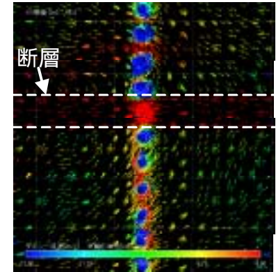
断層を想定したケースの透水係数場(左)およびダルシー流速分布(右)
