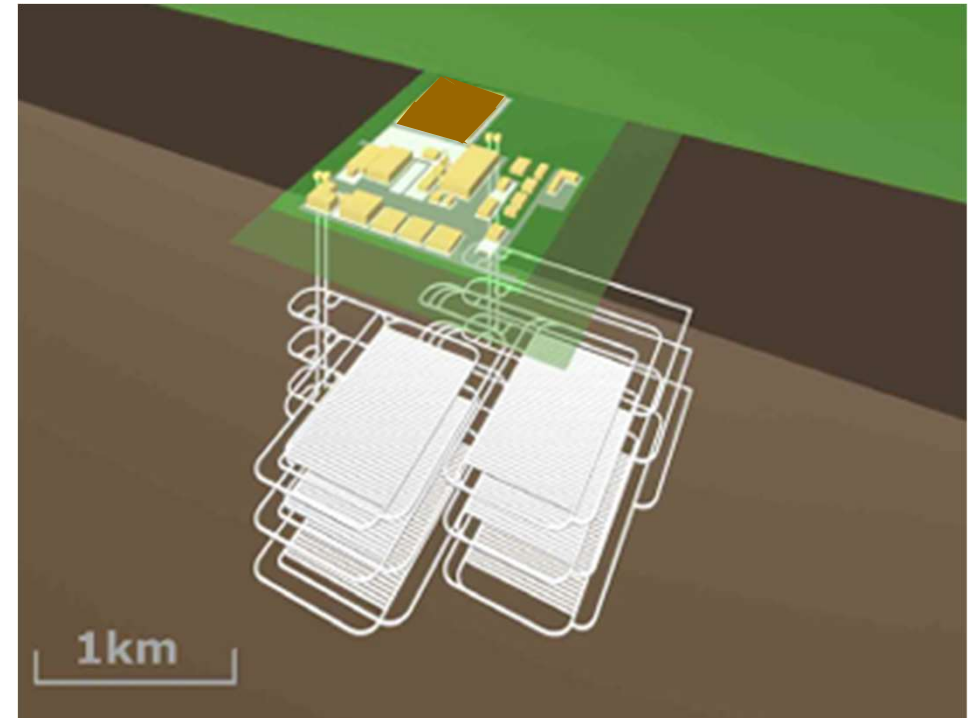
複層（3階建）レイアウトのイメージ
