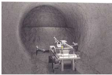
坑道の掘削
