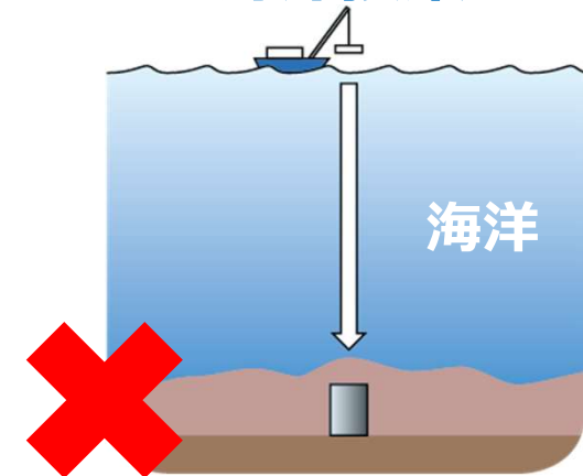
海洋投棄
