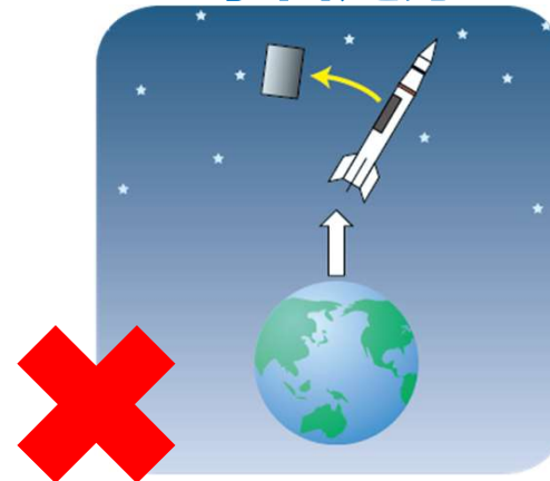
宇宙処分
