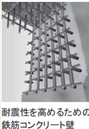
地震・津波
