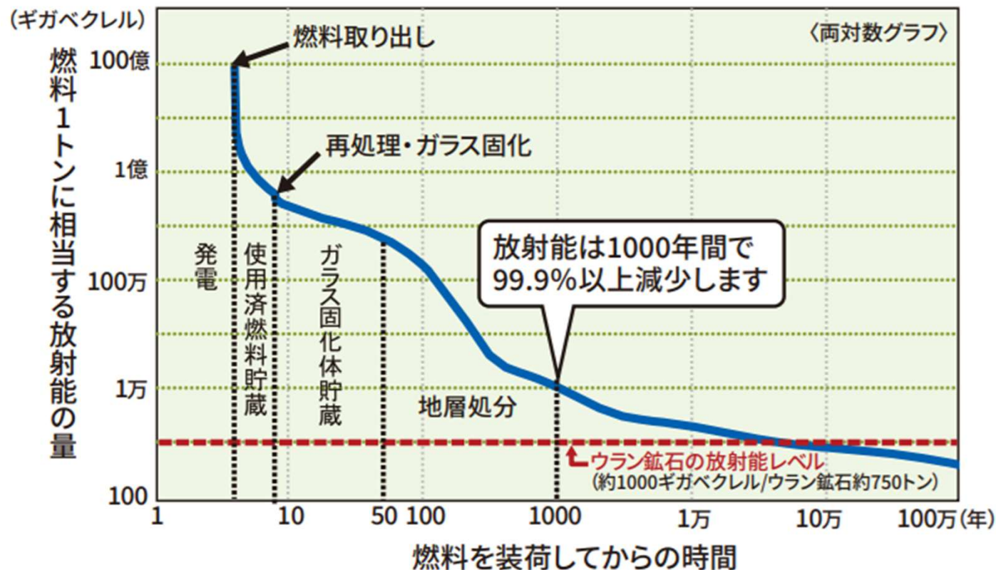
▼ ガラス固化体の放射能の経時変化
