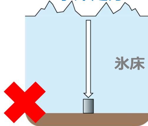
氷床処分
