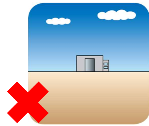
地上保管
