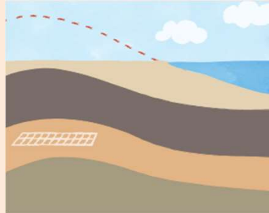
隆起・侵食
