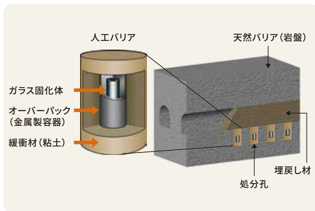
展示:地層処分実規模試験施設
