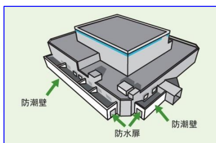
津波時の地上施設への浸水防止策
