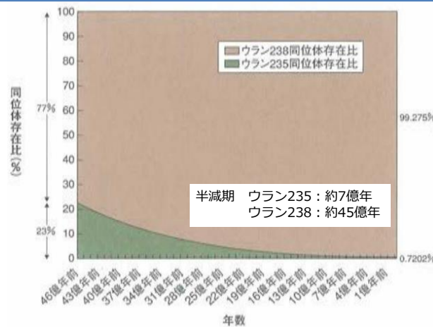
地球のウラン同位体存在比
