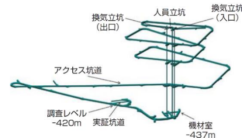
オンカロのレイアウト図
