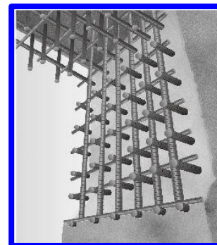
耐震性を高めるための 鉄筋コンクリート壁
