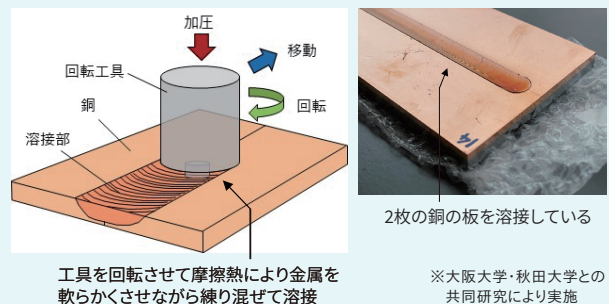
【図3】 摩擦熱による溶接の様子（左）と溶接部の外観（右）
