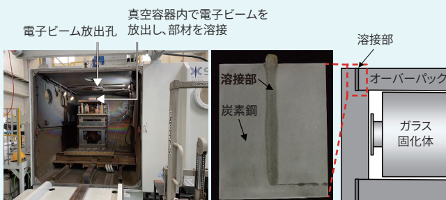
【図2】 電子ビームによる溶接機（左）と溶接部の断面（右）
