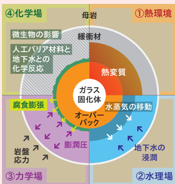
【図1】 処分場閉鎖後、人工バリアに生じる熱-水-応力-化学の複合的な現象
