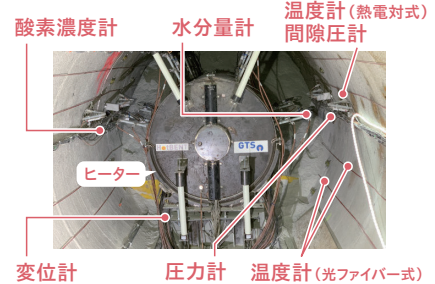
【図2】 スイスの地下研究所で実施している国際共同研究による実規模試験
