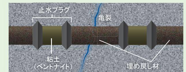
▲ 止水プラグの例
