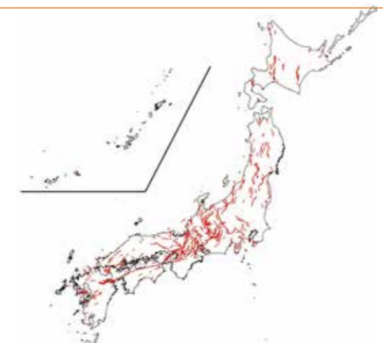
出典: 活断層データベース (産業技術総合研究所 https://gbank.gsj.jp/activefault/index_gmap.html )
