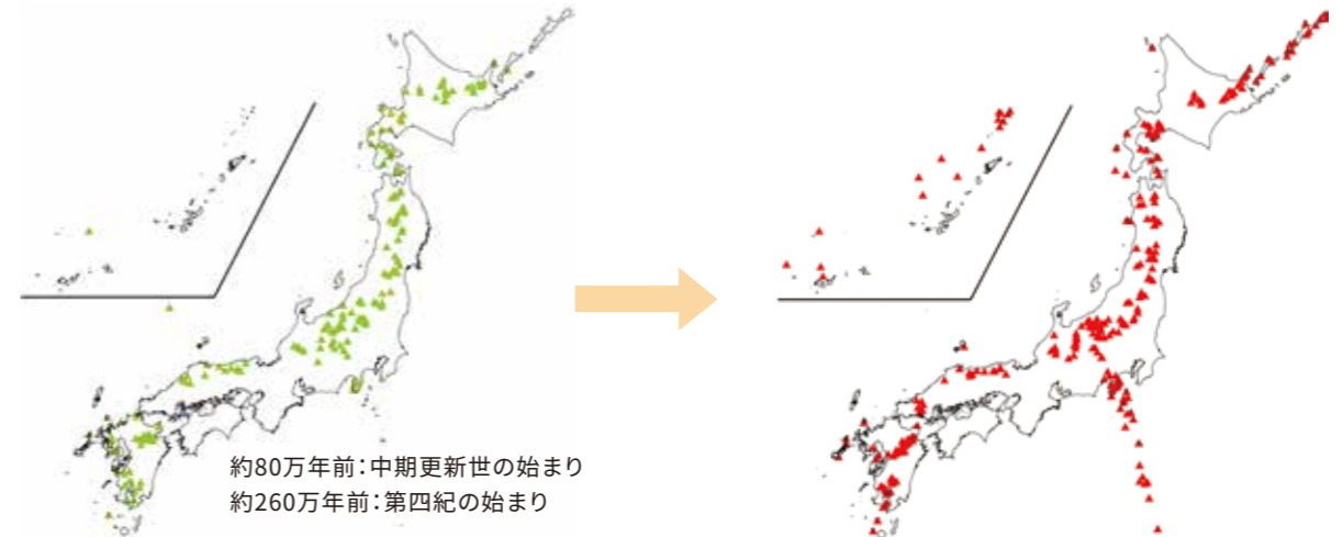
約80万年前: 中期更新世の始まり 約260万年前: 第四紀の始まり ・中期更新世とは: 第四紀の中の更新世(約260万年前から約1万年前)のうち、約80万年前から約13万年前までの期間 ・第四紀とは: 約260万年前以降の地質時代 日本の火山(第3版)(産業技術総合研究所地質調査総合センター)に基づいて作成
