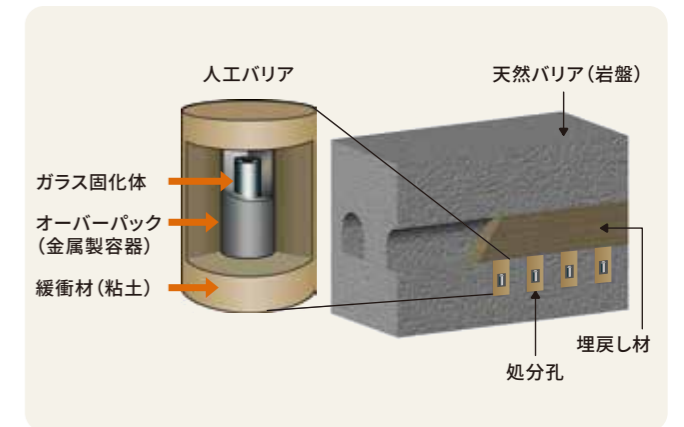
展示:地層処分実規模試験施設
