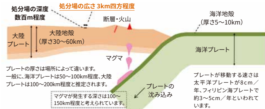
「地震がわかる!」(地震調査研究推進本部, 2017) (※) p.33を参考に作図。プレートの移動の速さ、地殻の厚さ及びマグマが発生する深さは、同資料のそれぞれp.25,30,33より。プレートの厚さは「プレート収束帯のテクトニクス学」(木村, 2002) p.12より。 (※) https://www.jishin.go.jp/main/pamphlet/wakaru_shiryo2/wakaru_shiryo2.pdf
