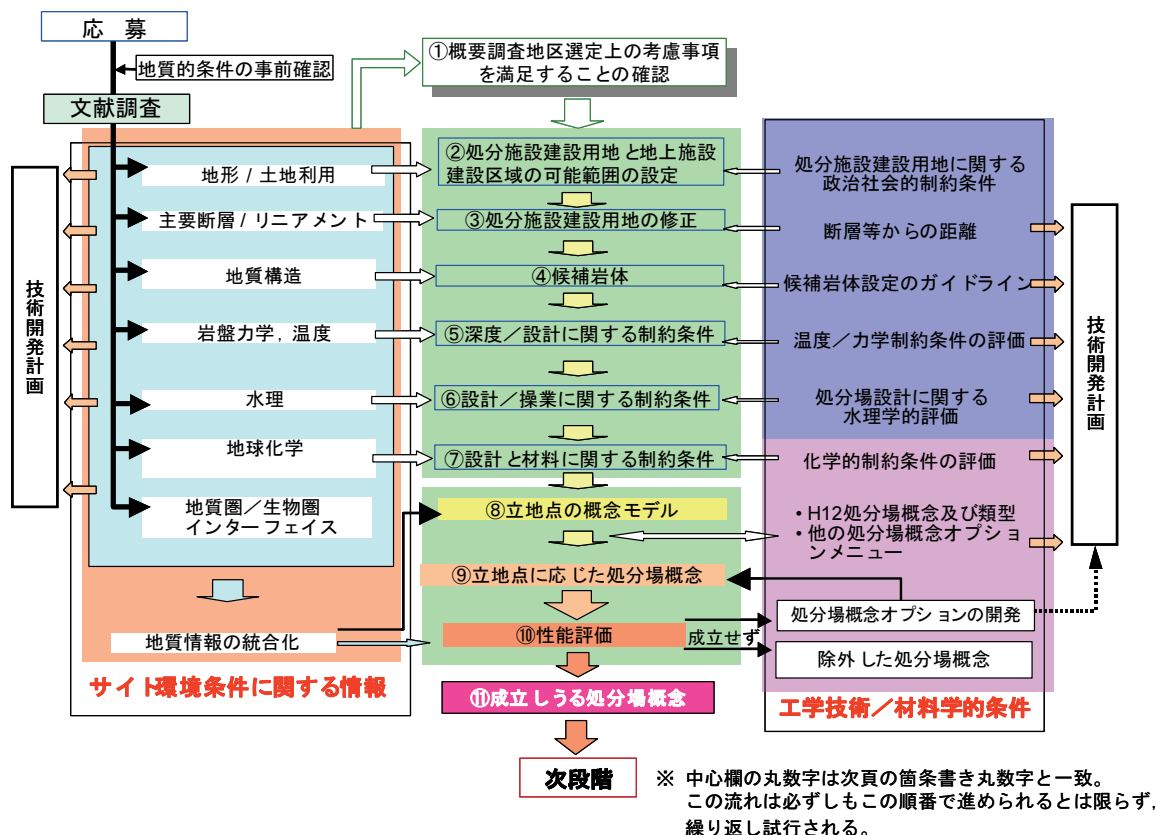
図 3.1-1 文献調査段階における処分場概念の検討の流れ (原子力発電環境整備機構，2004a を一部修正)
