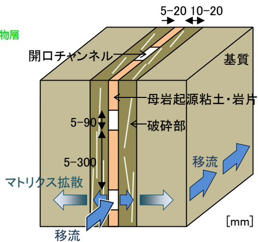
新第三紀堆積岩類
