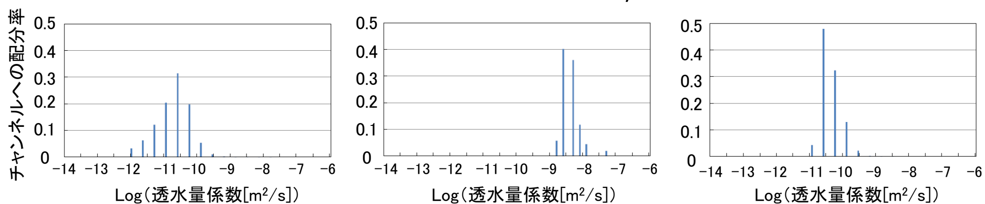
図-1 深成岩類
