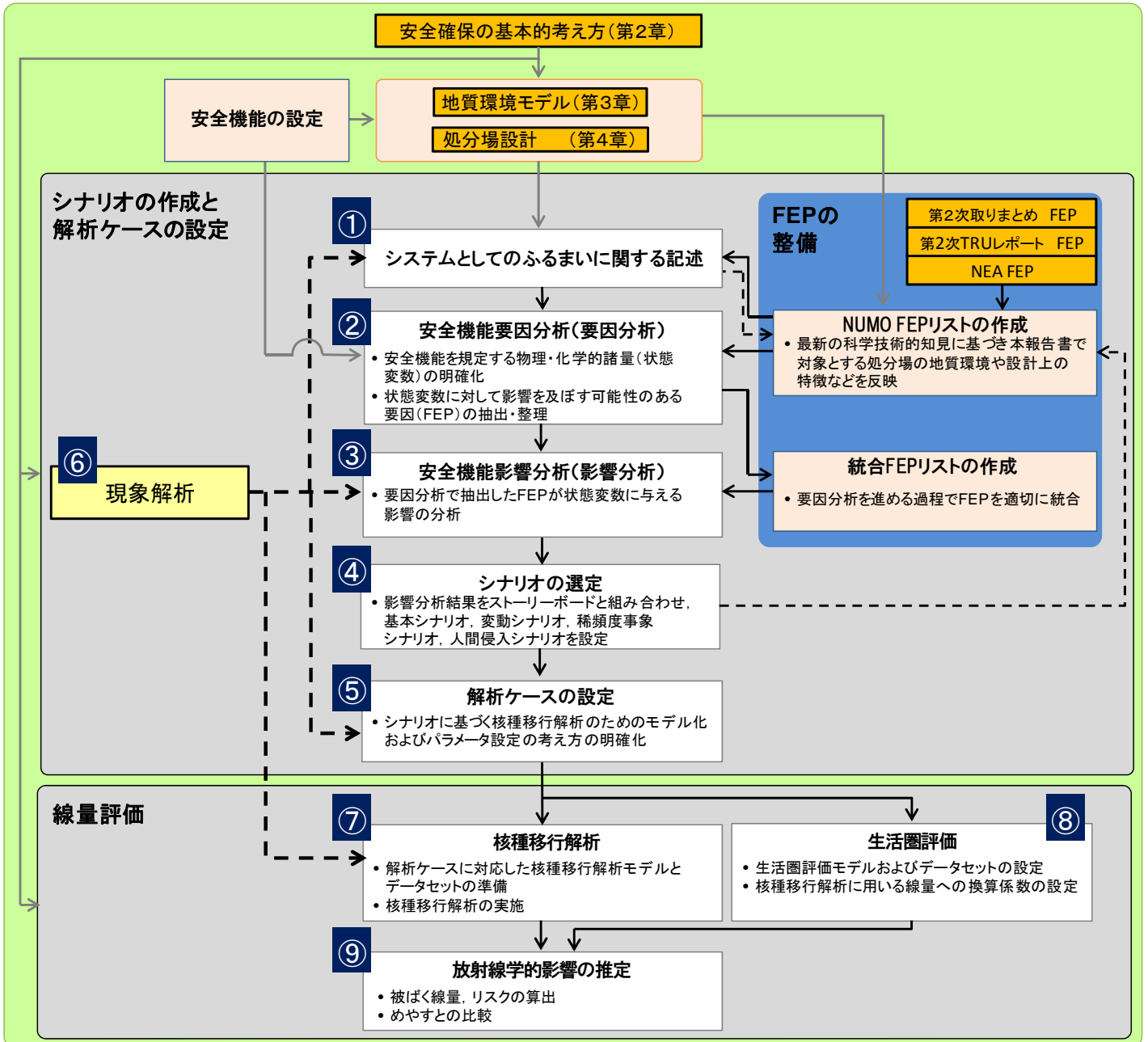
図-1 本報告書における安全評価の基本的手順
